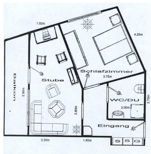
Grundriss Doppelzimmer
