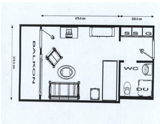
Grundriss Einzelzimmer
