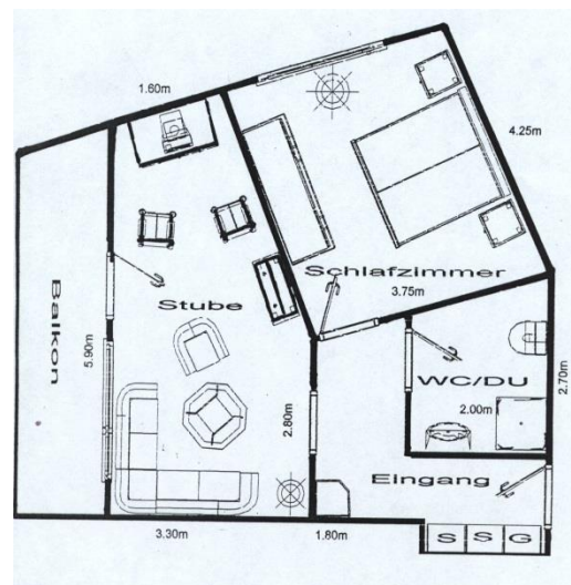
Grundriss Doppelzimmer
