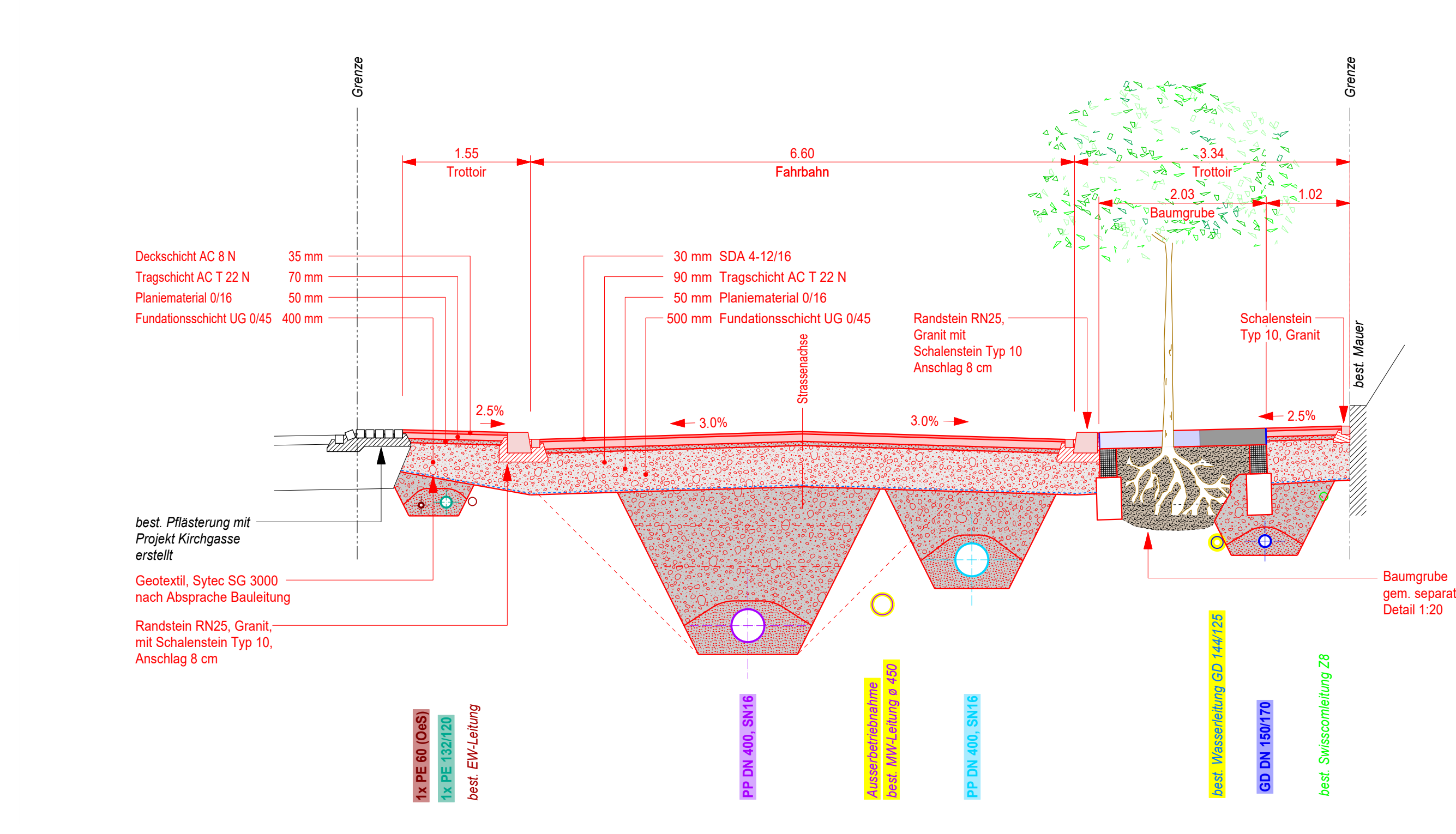
Normalprofil 6, 1:50
