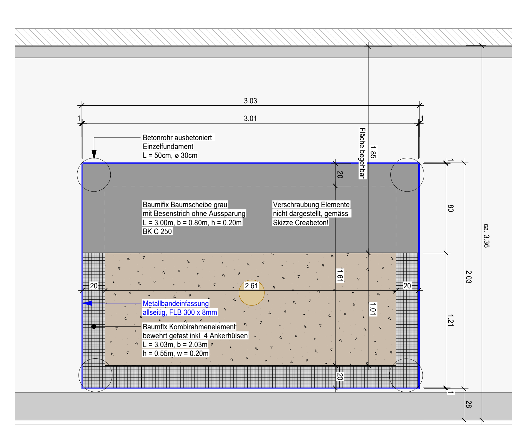
Detail Baumgrube Grundriss 1:20
