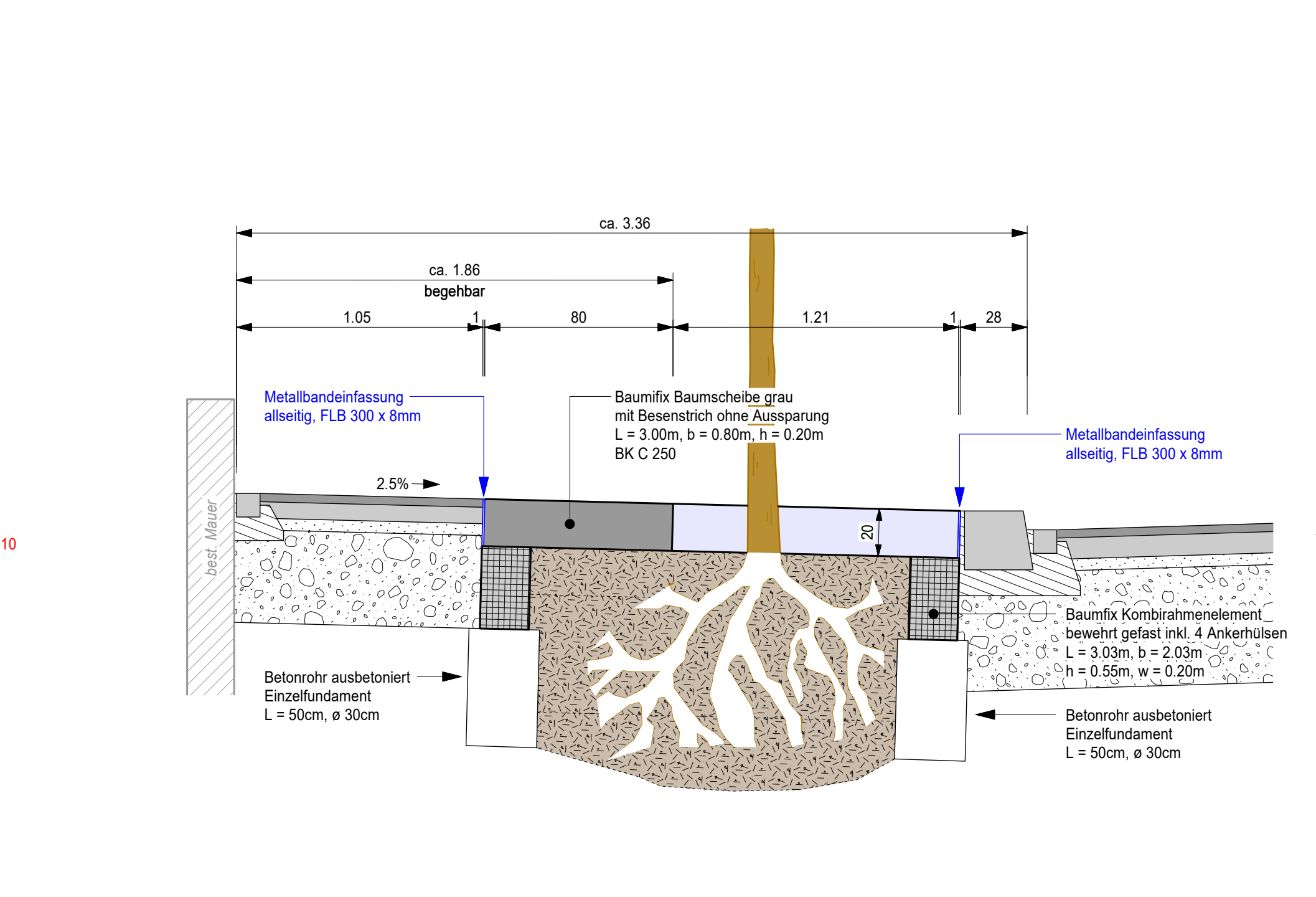
Detail Baumgrube Querschnitt 1:20
