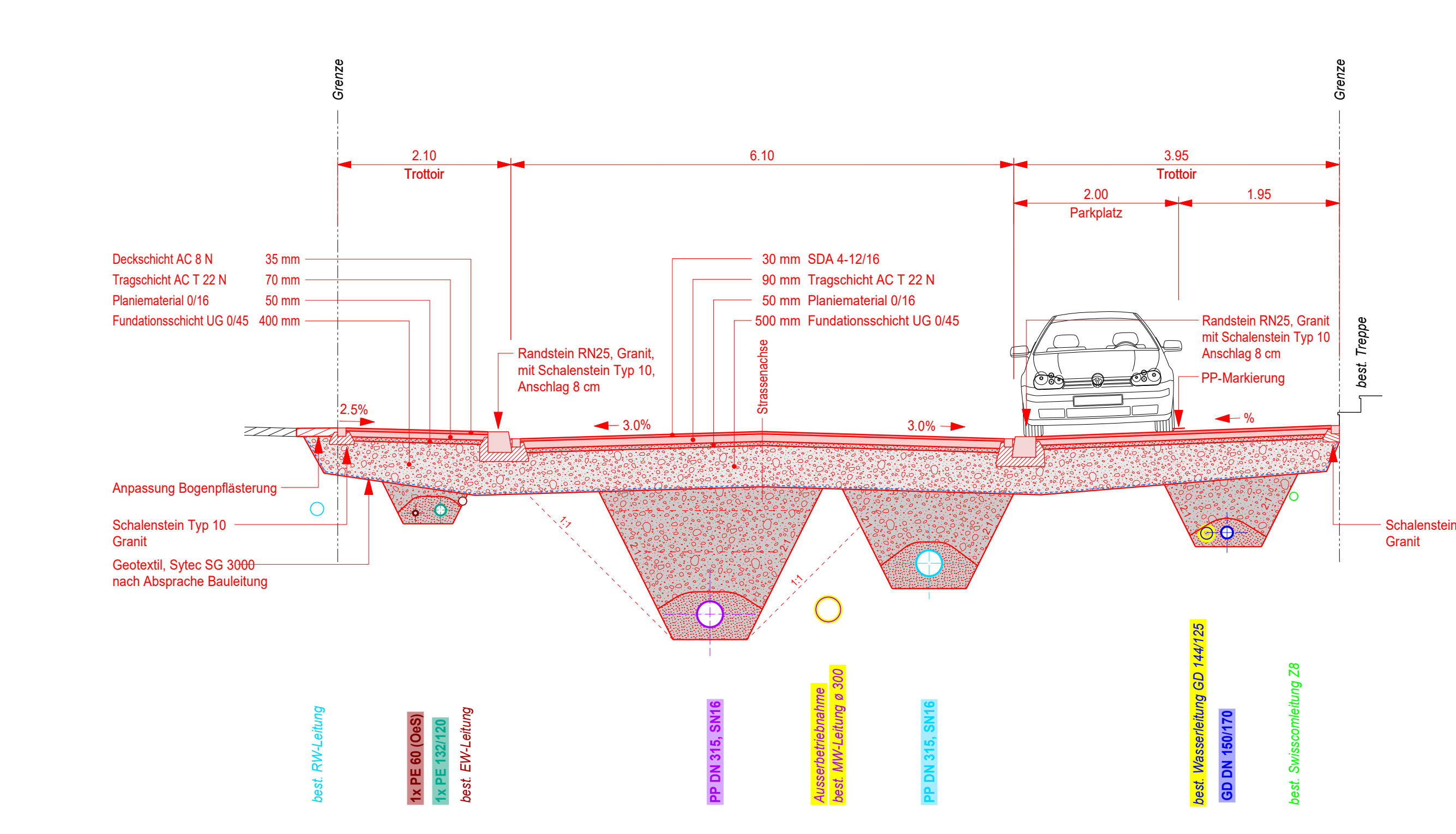
Normalprofil 7, 1:50
