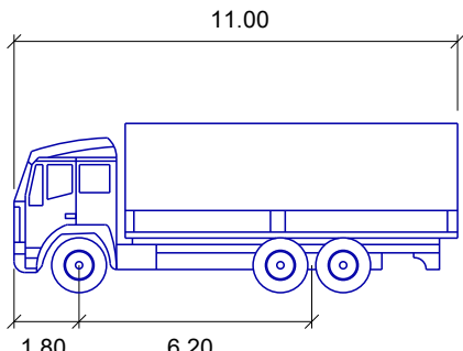
Lastwagen 11m Breite: 2.60m
